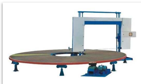
Автоматический комплекс карусельного типа для горизонтальной резки ППУ
