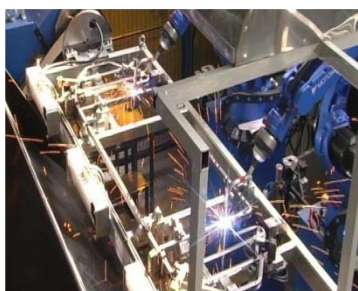
Сварочный робот
